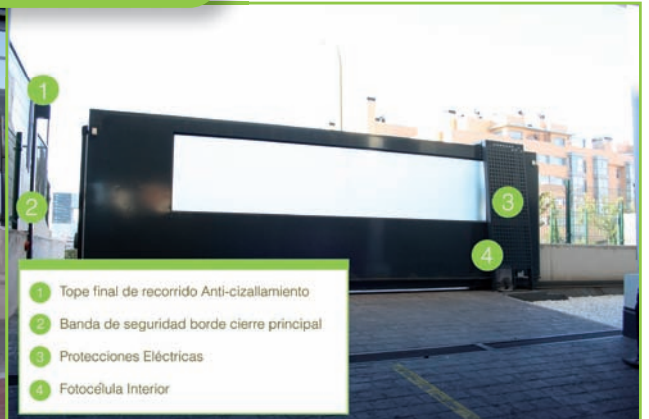
SEGURIDAD EN PUERTAS CORREDERAS | Vista Exterior/Interior
